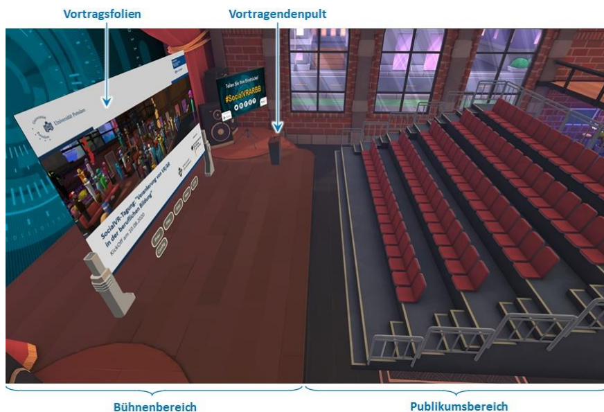
Abb. 1: Plenarsaal
